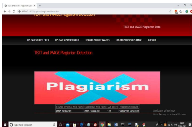
Fig. 13 LCS score
